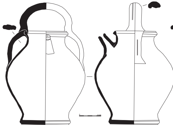
Pichet 401.070.027 (C. Romieu / Au. Vignet)
